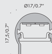
1:1 section tubino s sección 1:1 tubino s
