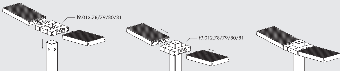
supporto palo doppio proiettore · double projector support pole f9.012.78/79/80/81
