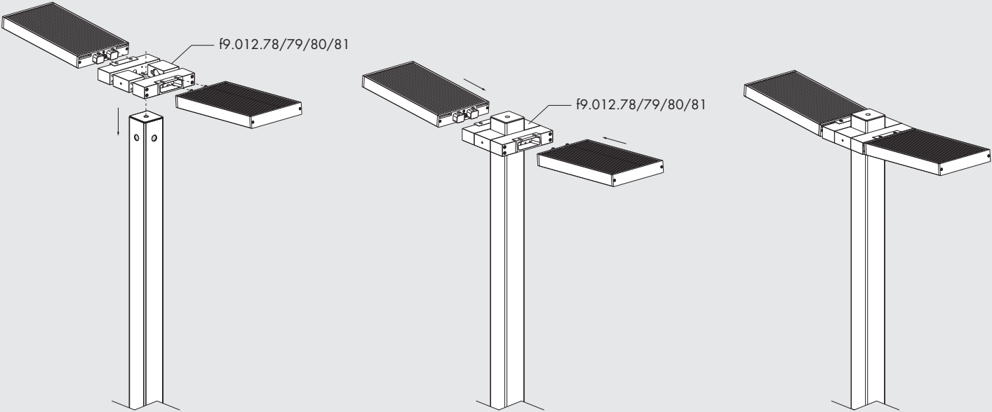
supporto palo doppio proiettore · double projector support pole f9.012.78/79/80/81
