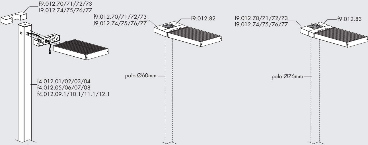
supporto palo singolo proiettore · single projector support pole f9.012.70/71/72/73
