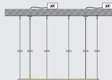
rosone di alimentazione a scomparsa totale · fully concealed rose
