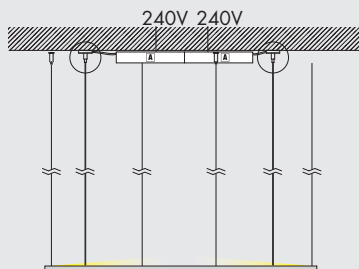
rosone di alimentazione soffitto · ceiling rose
