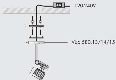
rosone con alimentatore remoto ceiling rose with remote power supply
