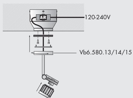
rosone con alimentatore remoto ceiling rose with remote power supply
