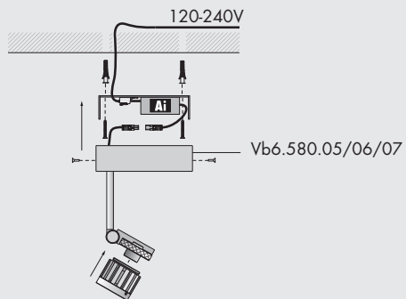
rosone con cassaforma laterizio per alimentatore ceiling rose with brick housing for power supply
