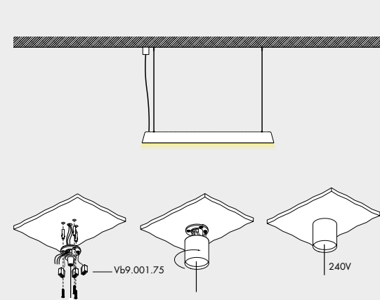
rosone di alimentazione · ceiling rose
