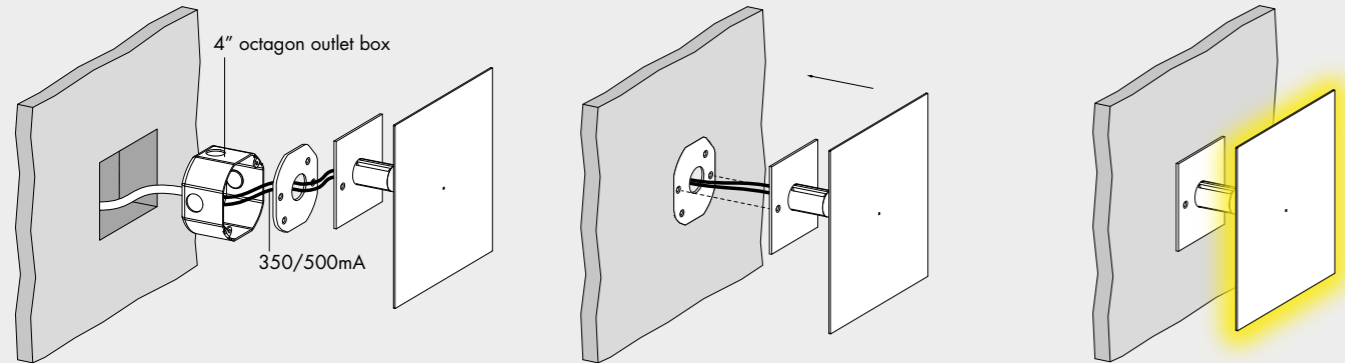
installazione con scatola modello usa/canada - installation with usa/canada outlet box
