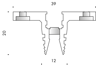
montantelettrico mb1 scala · scale 1:1
