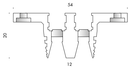
montantelettrico mb2 scala · scale 1:1
