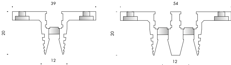
montantelettrico mb1 2000/3000mm scala · scale 1:1 montantelettrico mb2 2000/3000mm scala · scale 1:1
