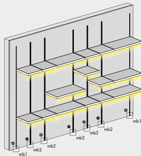
collegamento elettrico · electrical connection montantelettrico mb1
