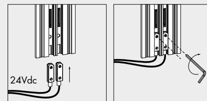
collegamento elettrico · electrical connection montantelettrico mb2
