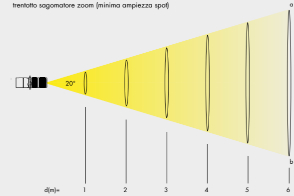
trentotto sagomatore zoom (minima ampiezza spot)
