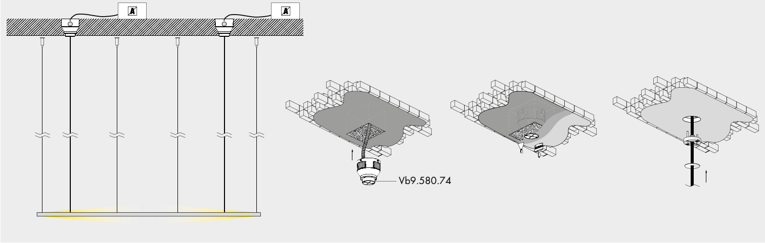
rosone di alimentazione a scomparsa totale · fully concealed rose
