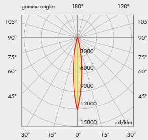
cilindro 58x160 13°
