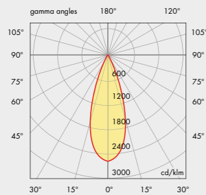
cilindro 58x160 36°
