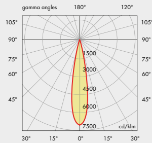
cilindro 58x160 20°
