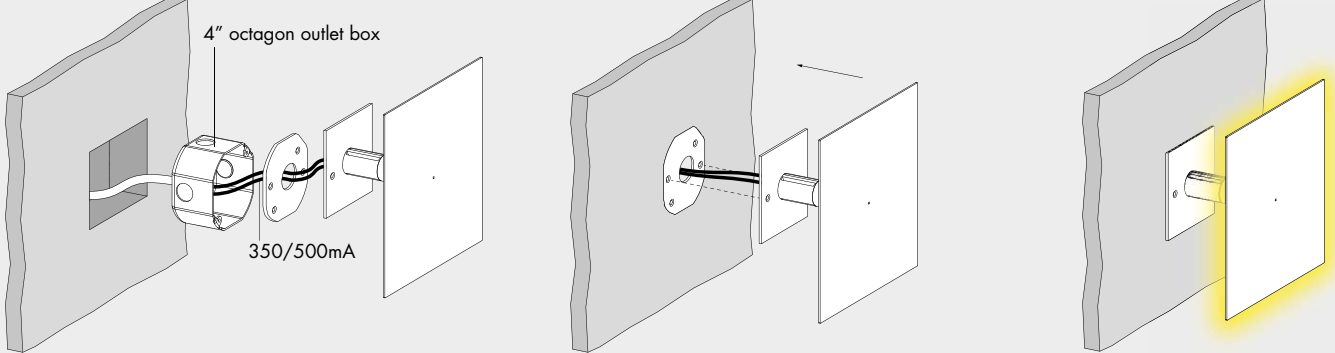
installazione con scatola modello usa/canada · installation with usa/canada outlet box
