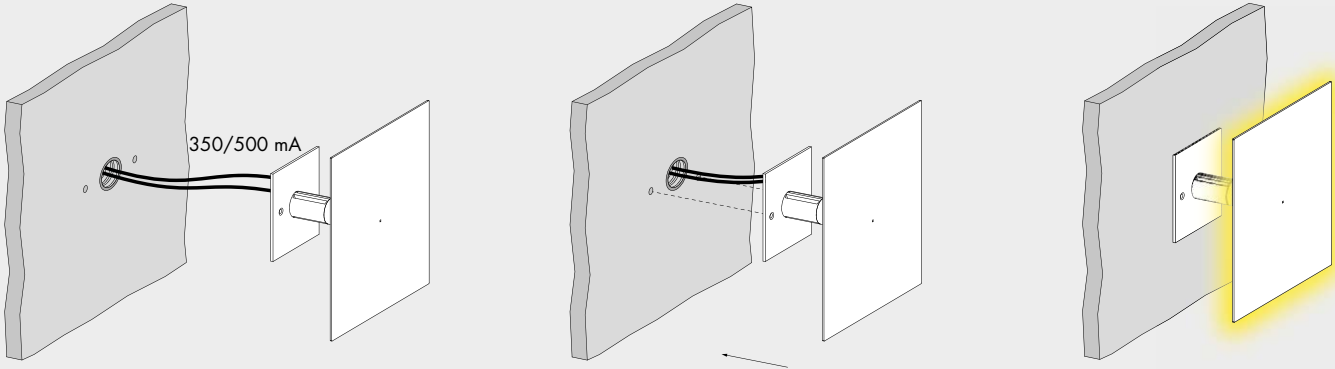
installazione con scatola incasso 3 moduli · installation with 3 modules recessed box
